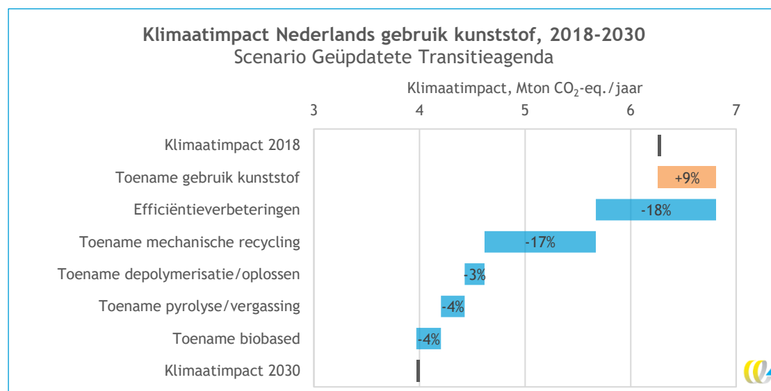
Figuur 9 - Ontwikkeling klimaatimpact Nederlands gebruik kunststof (productie, omzetting tot eindproducten en afdanking) tussen 2018 en 2030 in scenario Geüpdatete Transitieagenda, Mton CO 2 -eq./jaar
